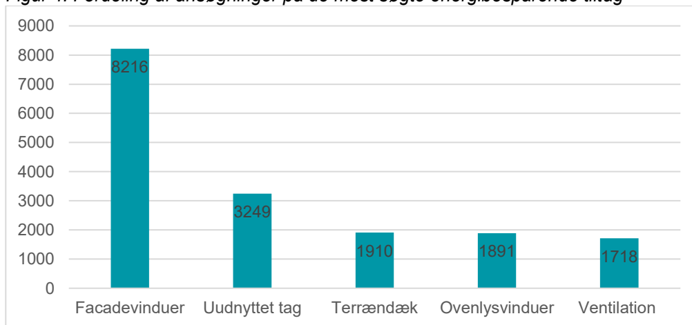
Figur 4: Fordeling af ansøgninger på de mest søgte energibesparende tiltag
